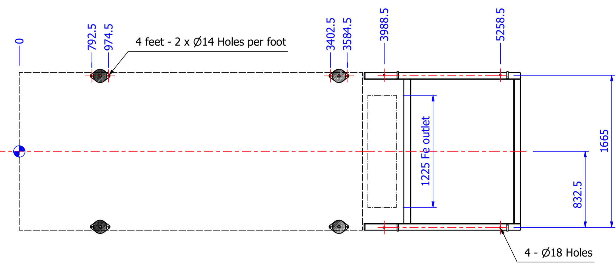
A-A ( 1 : 25 )
